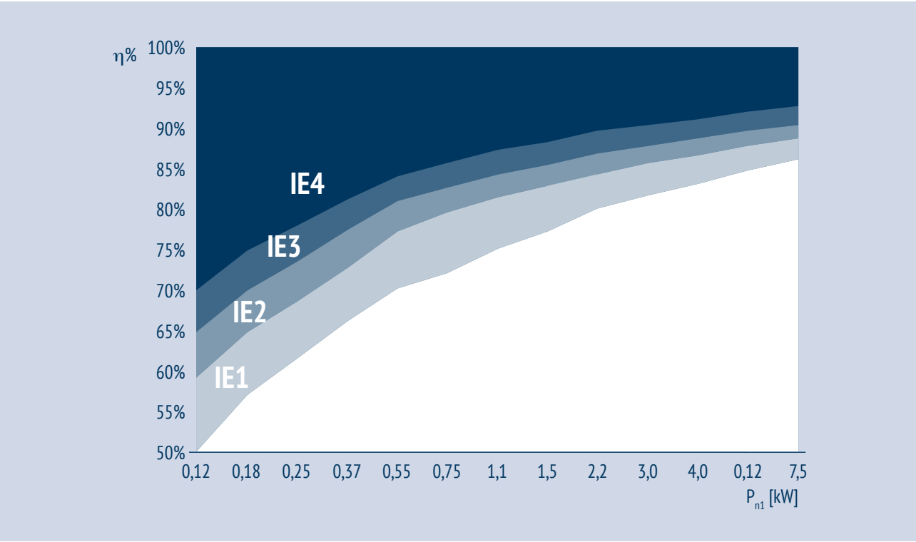
Classi di efficienza IE per motori a 4 poli a 50 Hz
