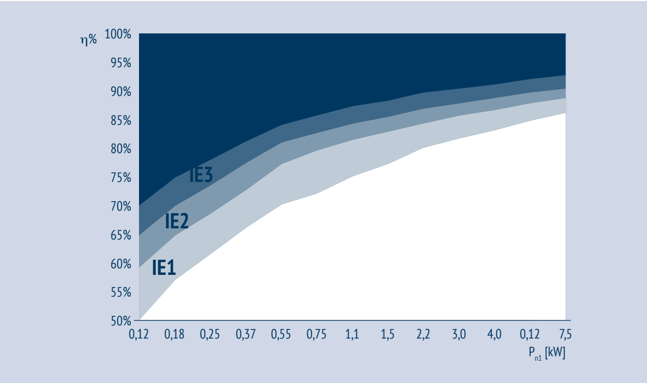
Clases de eficiencia IE para motores de 4 polos de 50 Hz
