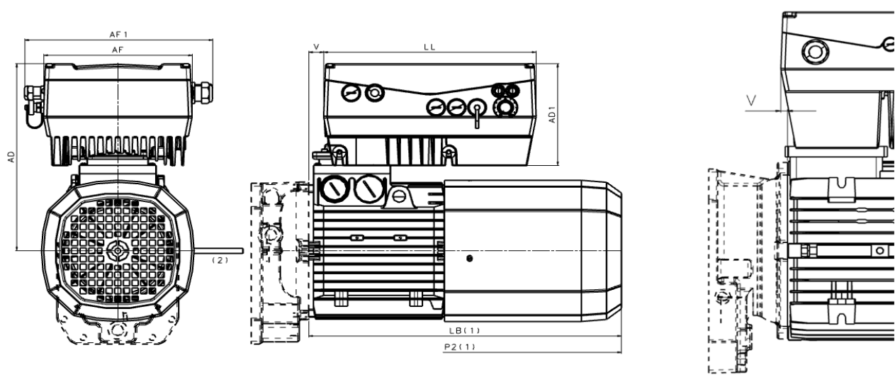
Moteurs : MX5
