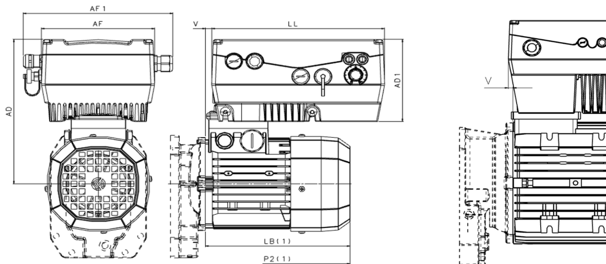
Moteurs : MX5
