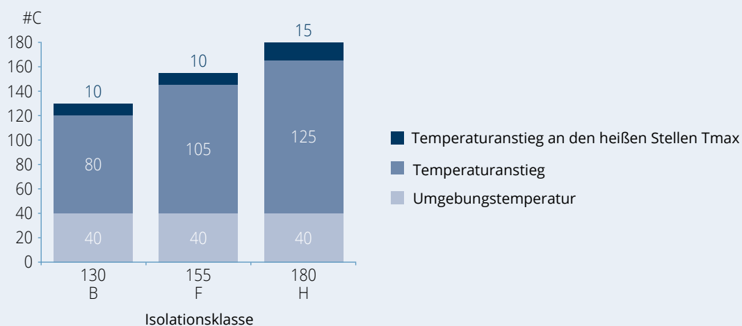
Temperaturanstieg (T) und Höchsttemperaturen an den heißen Stellen (Tmax) bei den Isolationsklassen (IEC 60034-1).
