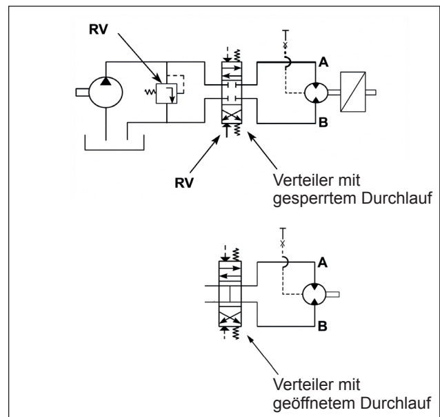
Offener Kreislauf
