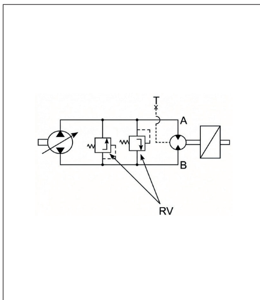
Geschlossener Kreislauf
