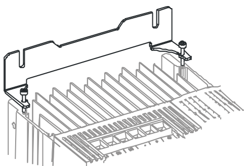
Befestigungswinkel oben (Befestigung mit Schrauben M4x20 )
