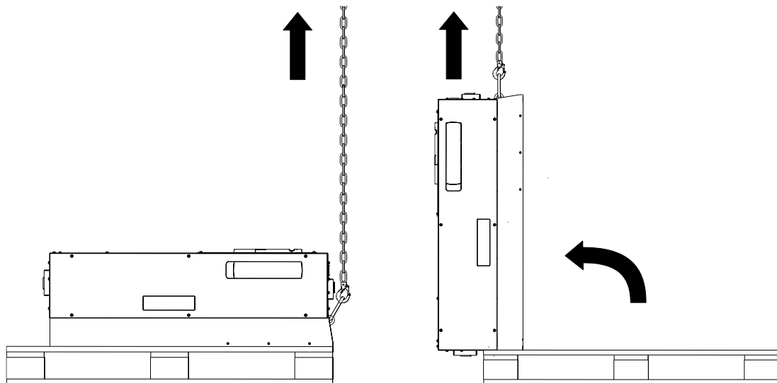
Abbildung 3-2: Anheben mit Kran
