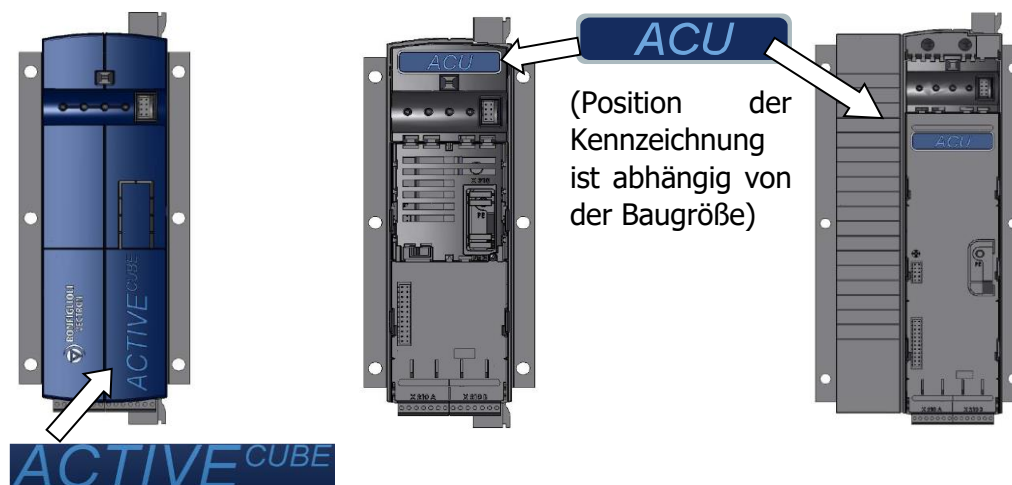
Abbildung 1-1: Gerätekennzeichnung
